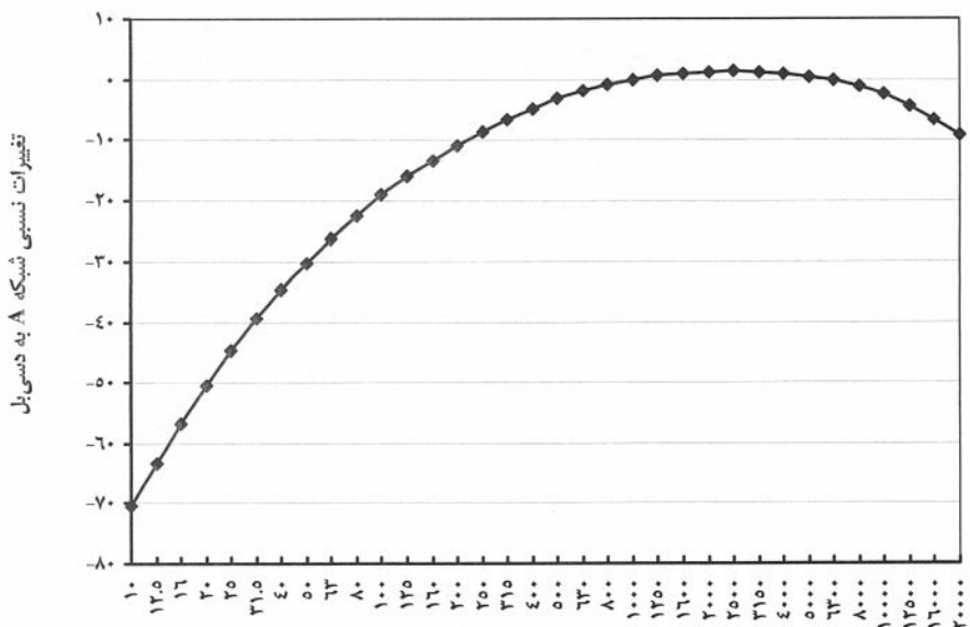
شکل ۱۸-۳-۱: نمودار تغییرات نسبی شبکه وزنی A در بسامدهای مختلف
