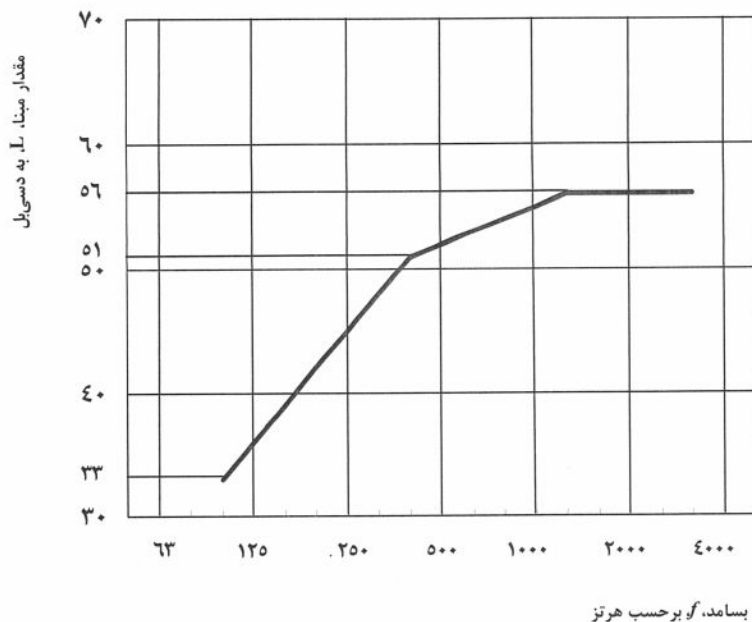
شکل ۱۸-۳-۱-۴: نمودار مقادیر مینا برای صدای هوابرد، در بندهای یک‌سوم هنگامی
