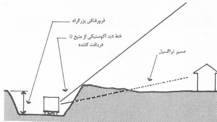
شکل پ-۵-۲: نمایش کاهش نوفه ترافیک توسط خاکریز طبیعی
