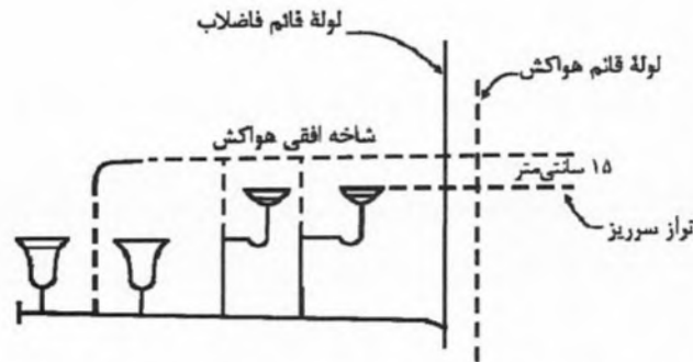
شکل ۱۶-۵-۲-۵ پ"۲- (۲) - اتصال هواکش به شاخه افقی لوله فاضلاب
