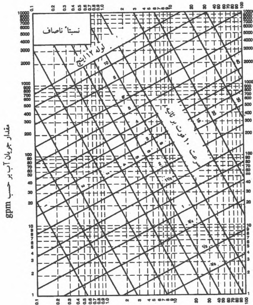
اقت فشار آب بر حسب فوت بر اینچ مربع در ۱۰۰ فوت طول
