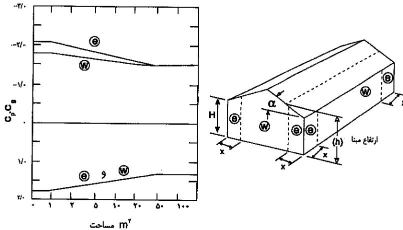
شکل ۶-۱۰-۵ ضرایب ترکیبی فشار و مکش خارجی C_{p,gs} برای طراحی دیوار و پوشش نما
